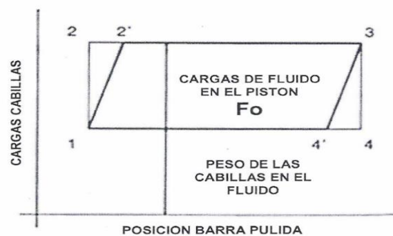
Fig. 2. Carta Dinagráfica de Superficie a diferentes velocidades de bombeo
